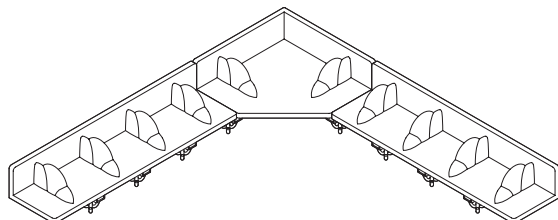
Wandgarderobe mit Mützenablage Wall coat and hat rack 33.7400.P9M 800-5200 x 800-5200 | 248 | 198
