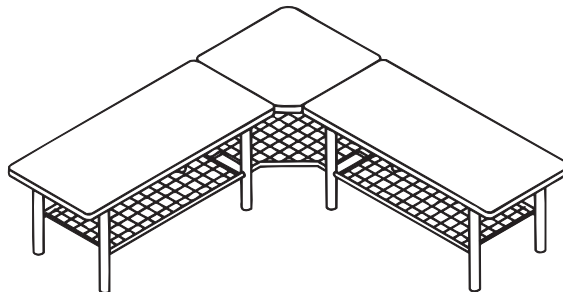
Sitzbank mit Schuhablage Bench with shoe rack 33.7441 1200-5200 x 1200-5200 | 340 | 350
